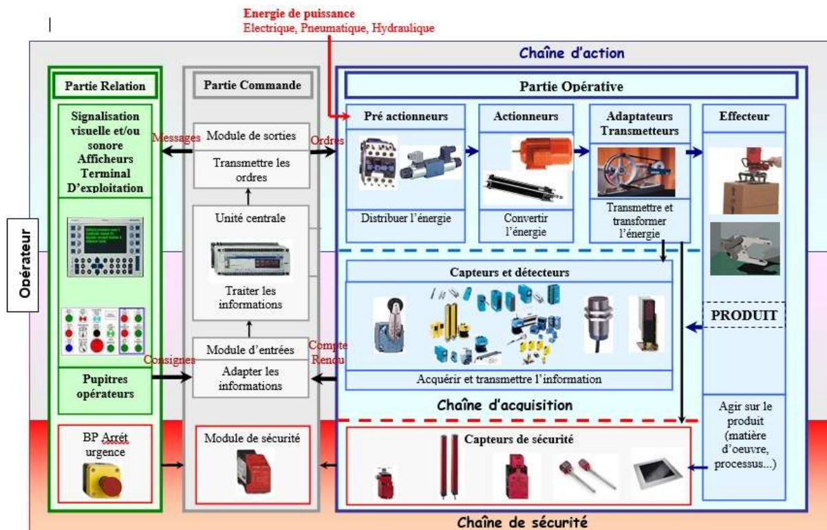
Figure 1 .2 : Schéma de principe d'un système automatisé de production
