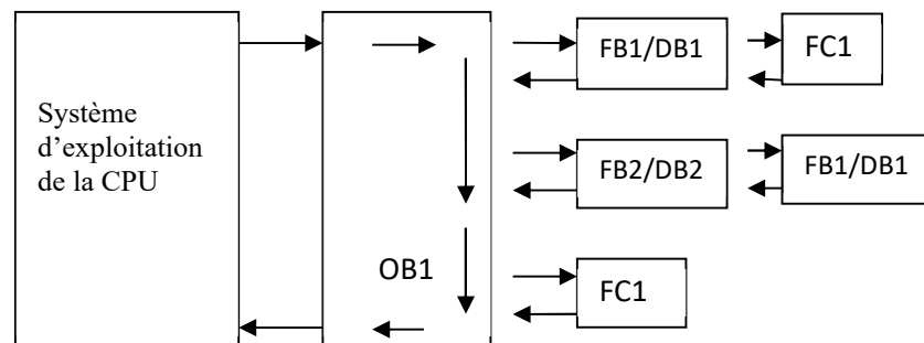
Figure 3- 13: Déroulement du programme principal dans la CPU
