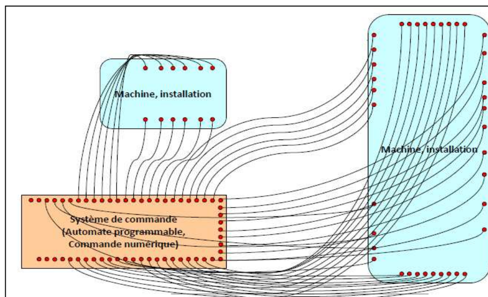
Figure 1 .4 : Schéma de principe d'une architecture centralisée
