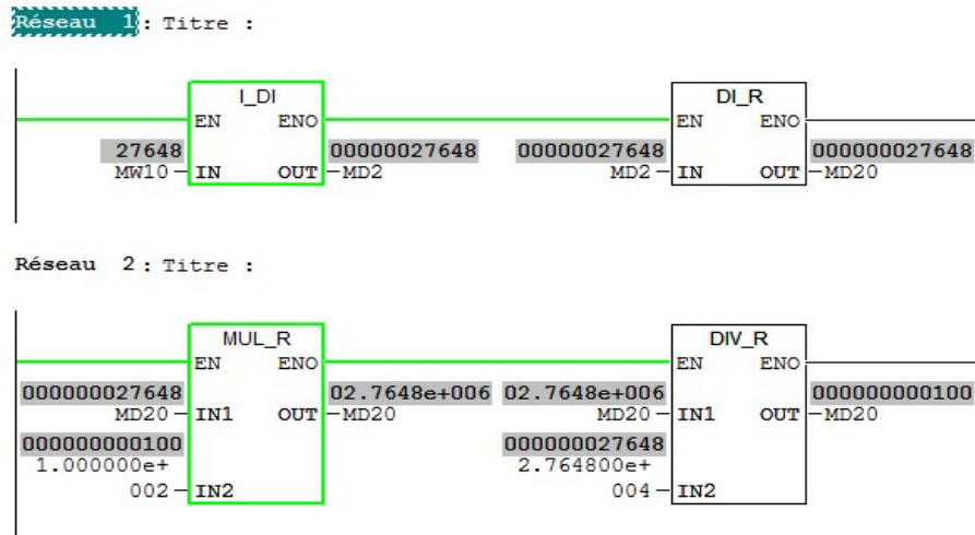
Figure 3- 29: Exemple de programmation d'une mise à l'échelle d'une entrée de type entier en format unipolaire (Résultat de simulation pour MW10 = 27648)
