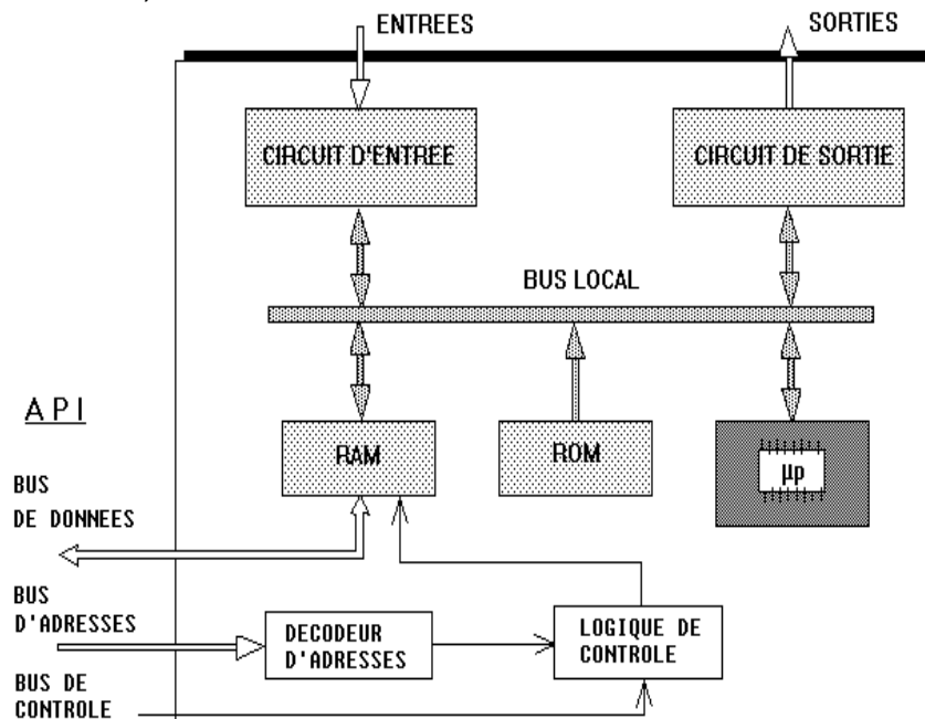
Figure 1-11: Schéma fonctionnel des modules d'entrées / sorties complexes
