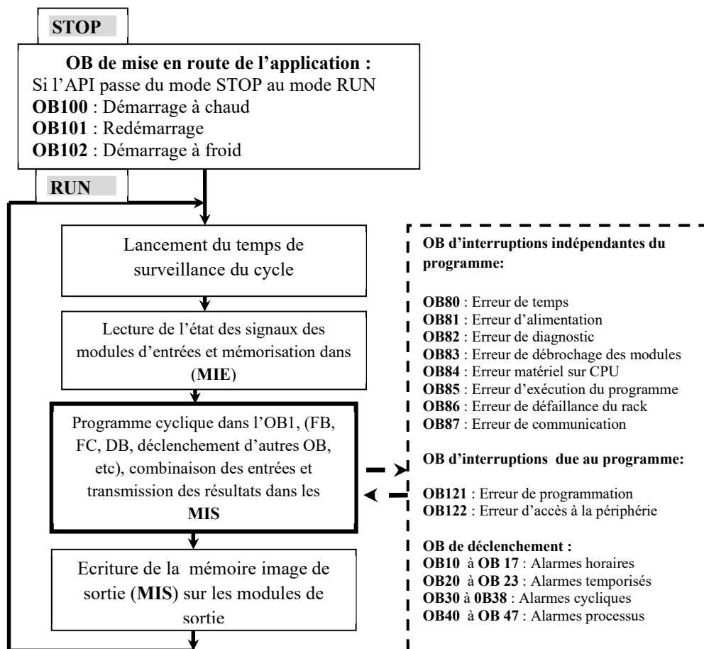
Figure 3- 12: Cycle de déroulement d'un programme dans la CPU
