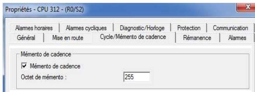
Figure 2- 7 : Configuration du memento de cadence lors de la configuration de la CPU
