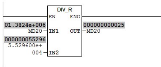
Figure 3- 32: Exemple de programmation d'une mise à l'échelle d'une entrée de type entier en format bipolaire (Résultat de simulation pour MW10 = -13824)
