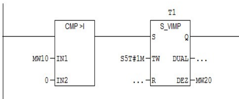
Figure 3- 47: Programme de déclenchement de la temporisation
