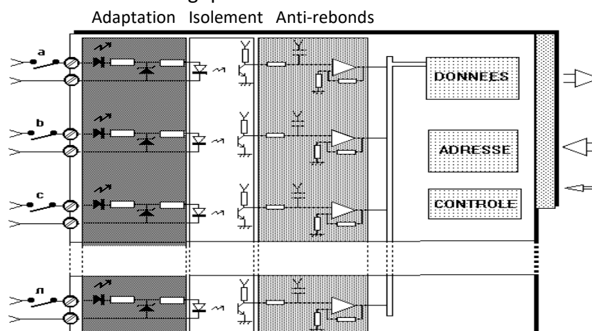
Figure 1-8: Eléments de base d'un module d'entrées logiques
