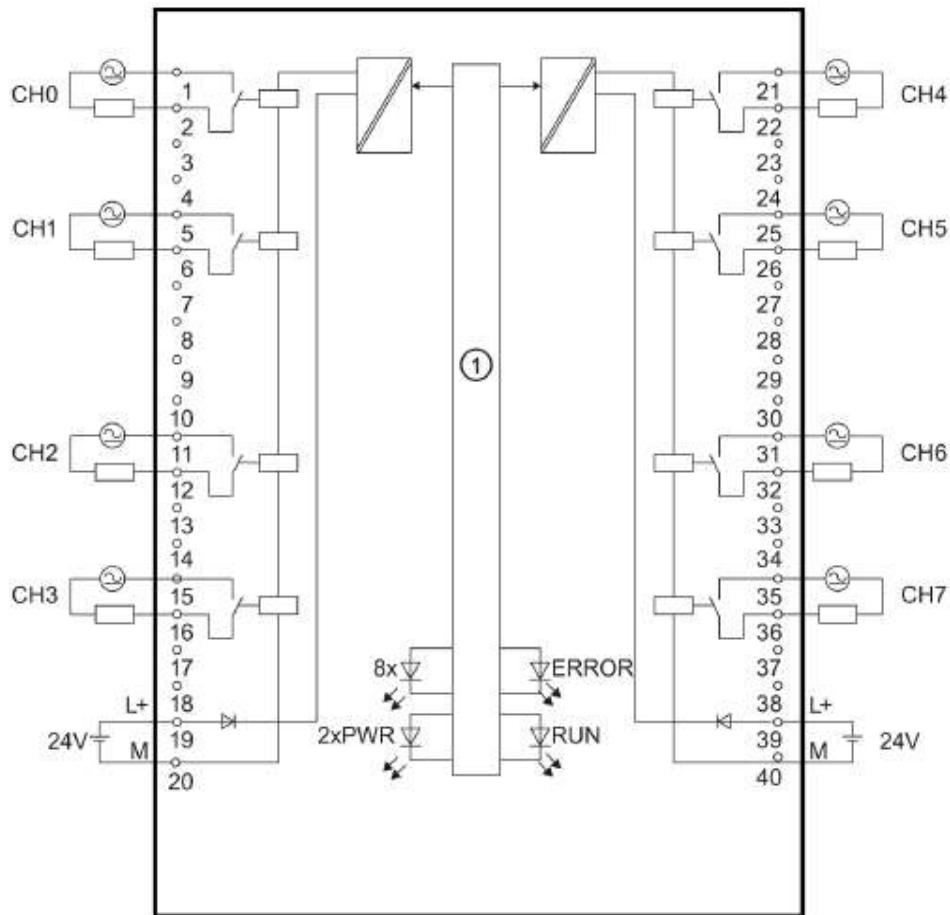
Figure 1.34 : Schéma de câblage d'un module de sortie logique à relais – (Module 8DQ à relais (6ES7 522 5HF00 0AB0))
