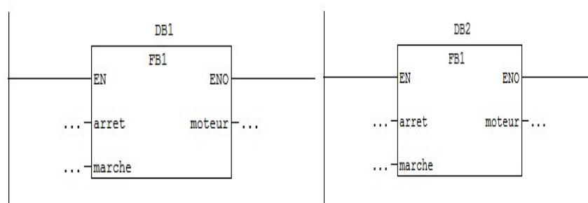
Figure 3- 22: Appel multiple à un bloc fonctionnel à partir de OB1
