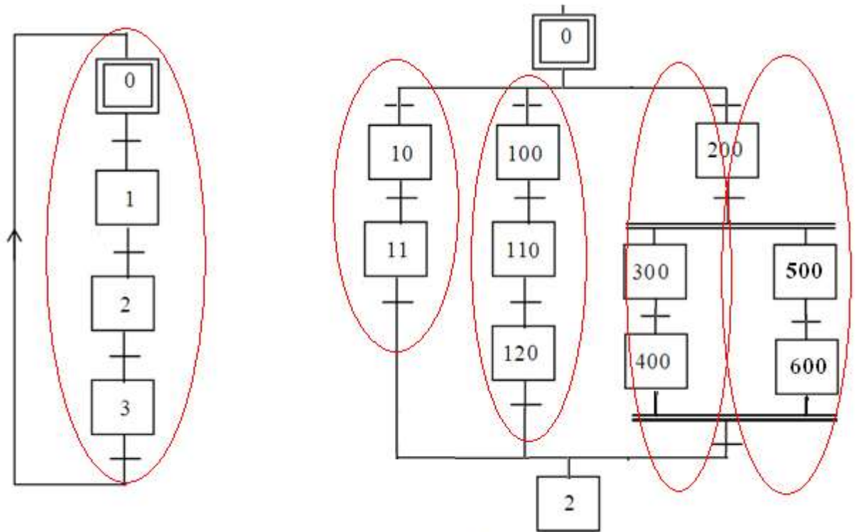
Grafcet à séquence unique.
