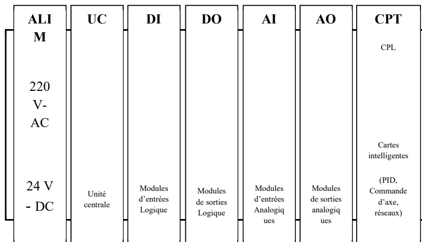
Figure 1 .6 : Exemple d'architecture matérielle d'un API
