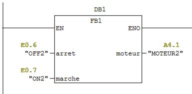
Figure 3- 21: Exemple d'appel à un bloc fonctionnel à partir d' OB1
