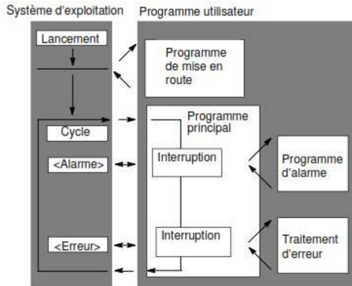
Figure 3- 9: Cycle de déroulement d'un programme dans la CPU
