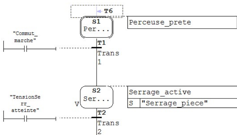
Figure 1-17: Exemple de programme écrit en langage GRAFCET
