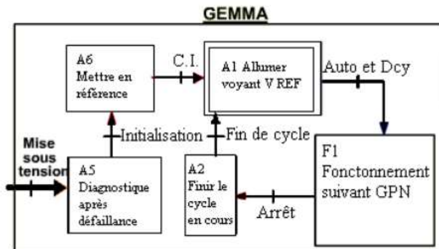
Figure 2.22 : Exemple de GEMMA d'un système.
