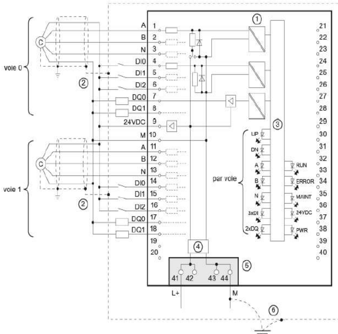
Figure 1.39 : Schéma de câblage du module TM Count 2x24V (6ES7 550 1AA00 0AB0).
