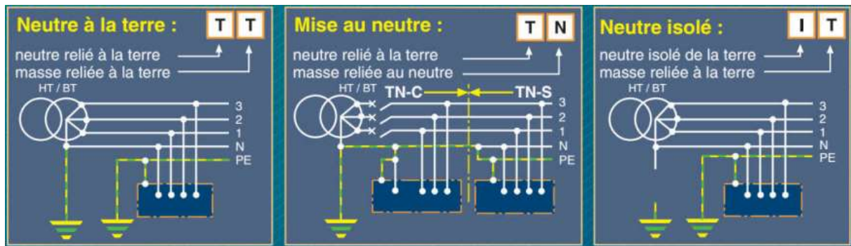
Figure 1-22: Schémas de branchement de l'alimentation d'un API selon le régime de neutre
