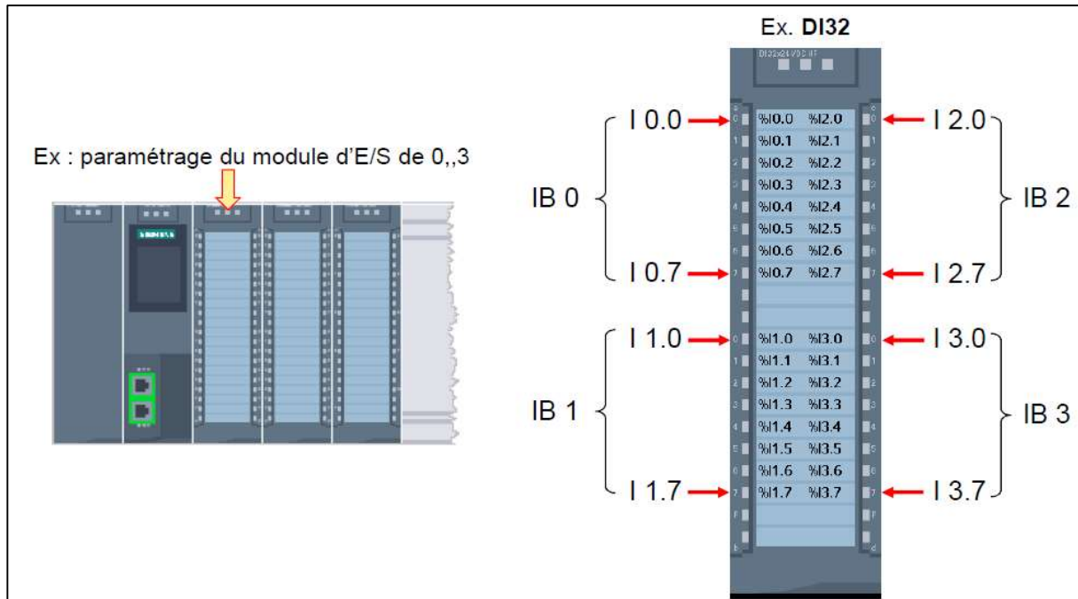
Figure 1.29 : Exemple d'adressage d'un module d'entrée logique DI32 de l'API S7-1500
