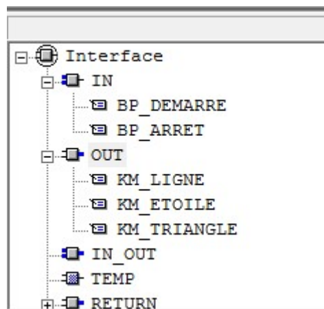
Figure 3- 40: Configuration des variables du bloc fonctionnel FC1
