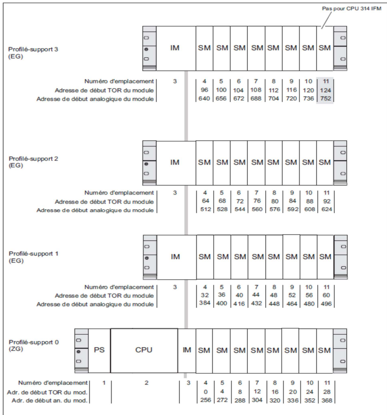
Figure 3- 3 : Emplacements du S7-300 et adresses initiales des modules correspondantes
