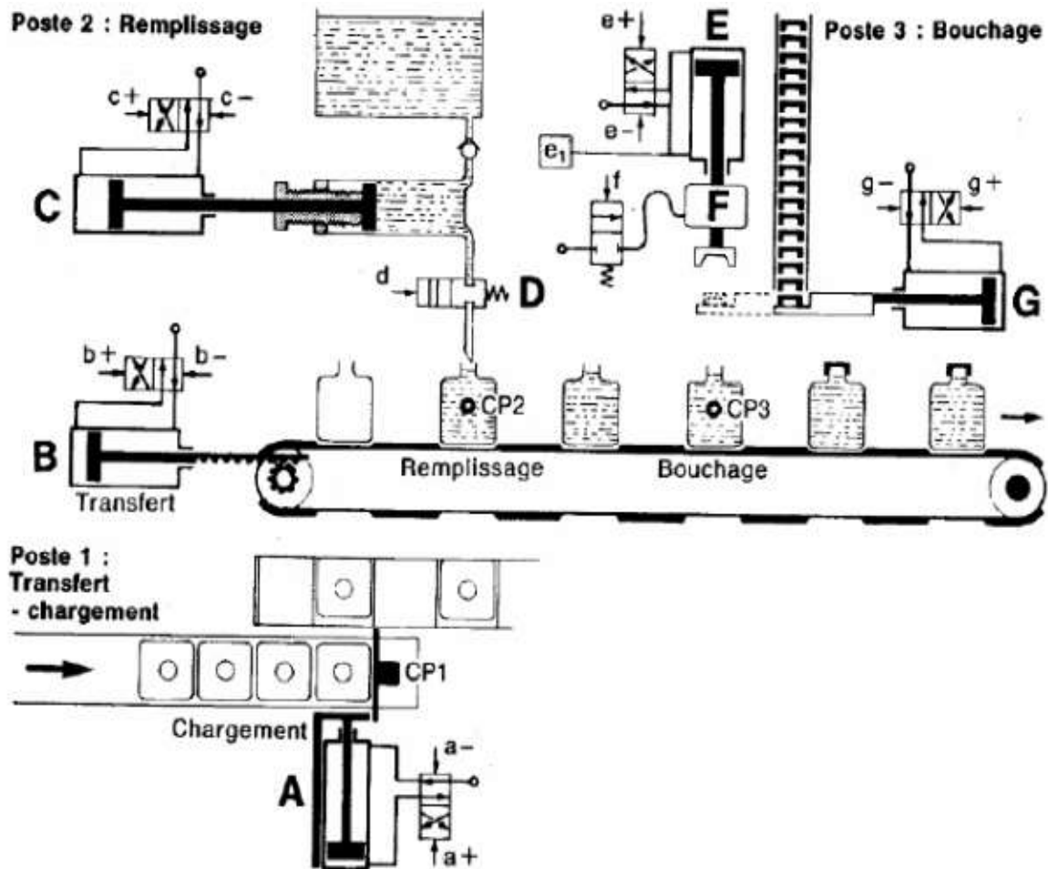
Figure 2.19 : Schéma de principe de la Machine à remplir et à boucher
