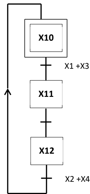
GRAFCET de tâche T1
