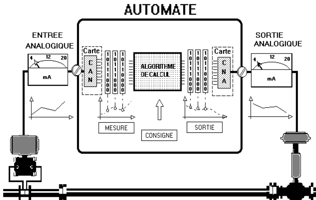
Figure 1-10: Schéma fonctionnel des modules d'entrées / sorties analogiques
