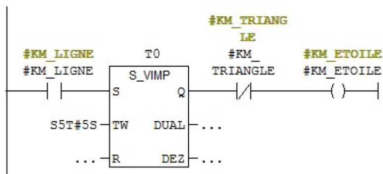
Figure 3- 42: Réseau de commande du contacteur (KM_Etoile)
