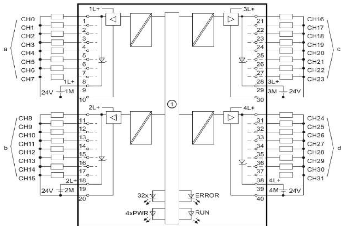
Figure 1.33 : Schéma de câblage d'un module de sortie logique à transistors - Module 32DQ (6ES7 522 1BL10 -0AA0)
