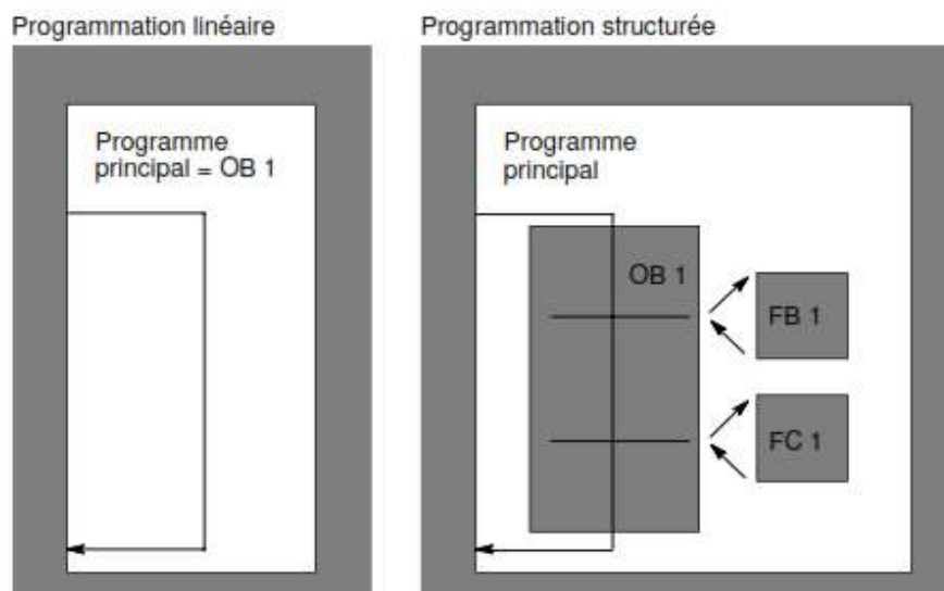
Figure 3- 10: Programmation linéaire et programmation structurée
