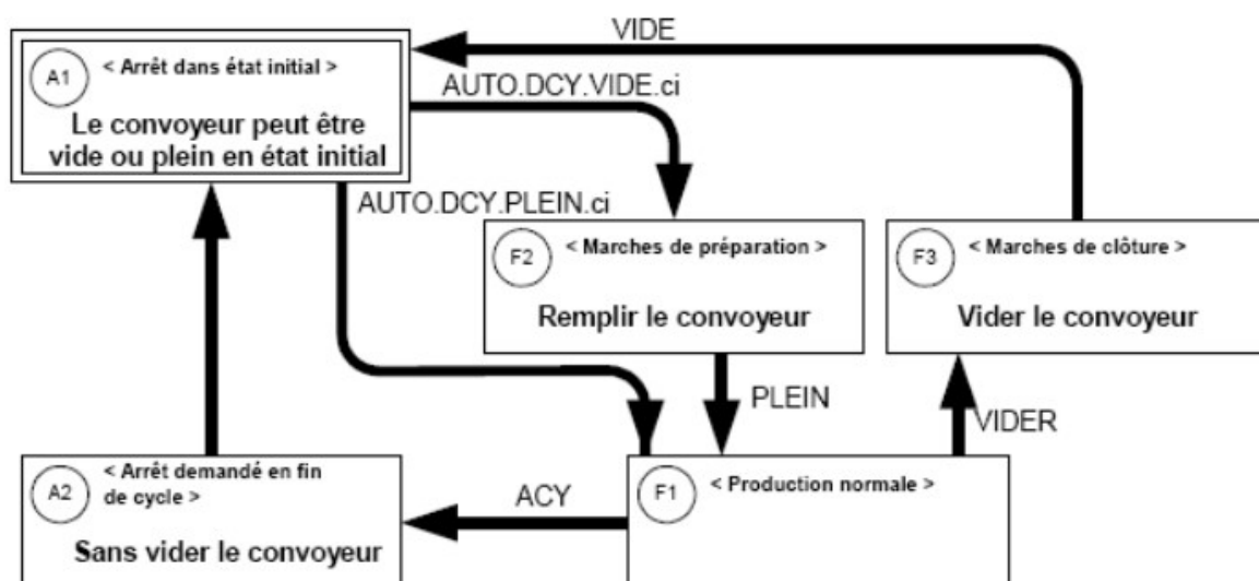
Figure 2.10 : GEMMA d'une machine avec marche de préparation et marche de clôture.
