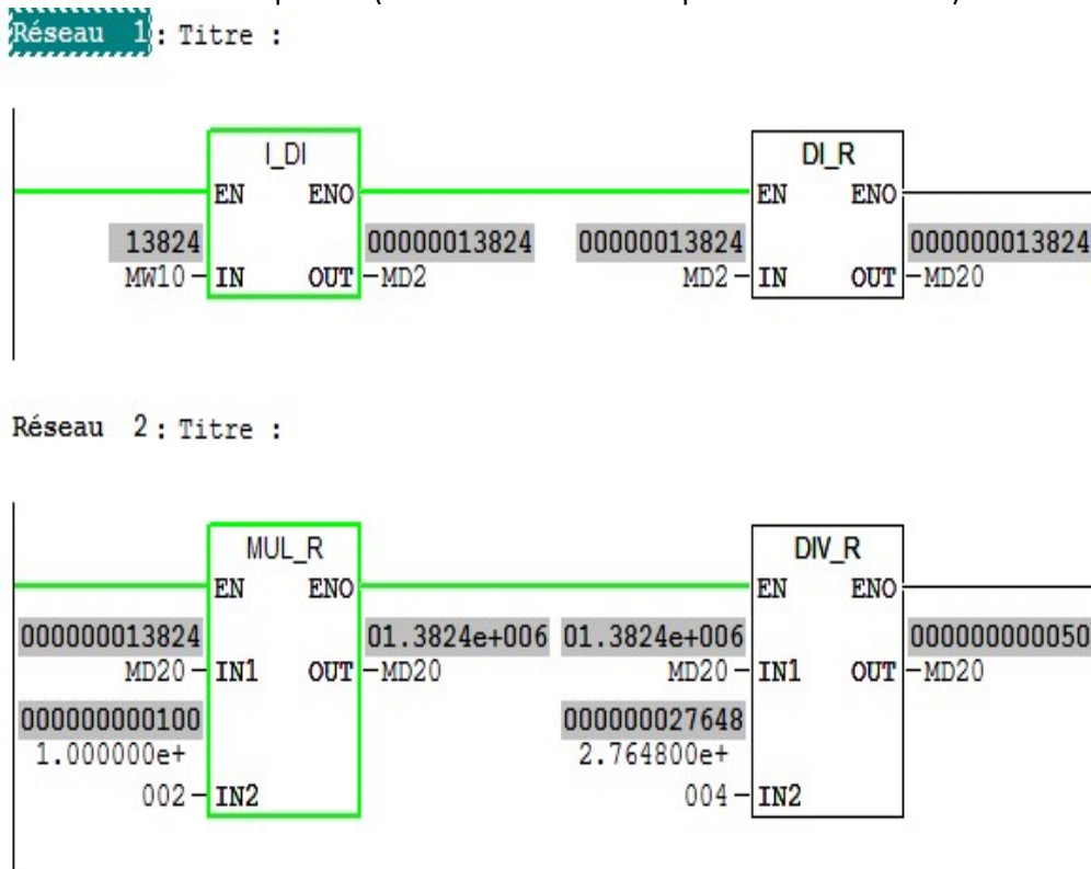
Figure 3- 30: Exemple de programmation d'une mise à l'échelle d'une entrée de type entier en format unipolaire (Résultat de simulation pour MW10 = 13824)
