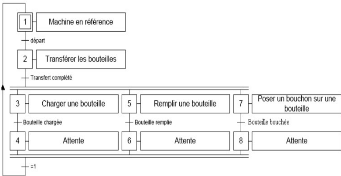
Figure 2.20 : (Grafcet niveau 1) de la Machine à remplir et à boucher
