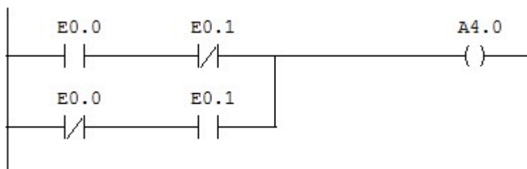
Figure 1-15: Exemple de programme écrit en langage ladder
