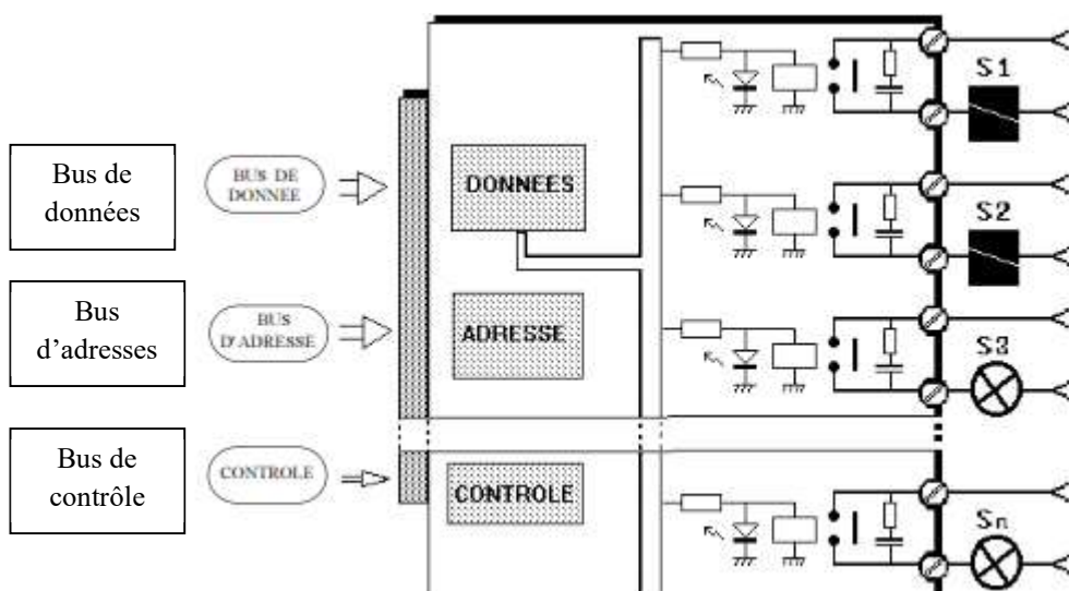
Figure 1-9: Eléments de base d'un module de sorties logiques à relais
