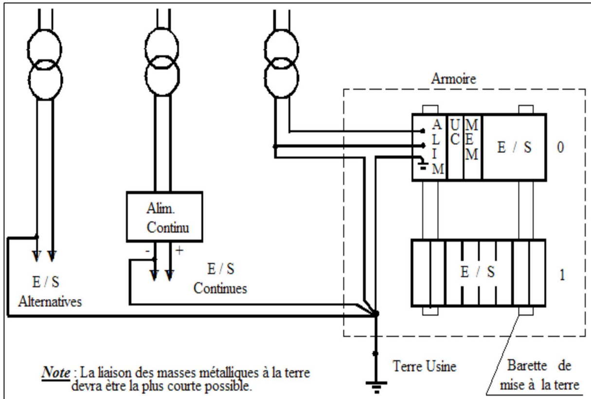
Figure 1-23: Schéma de principe de raccordement des alimentations d'une armoire
