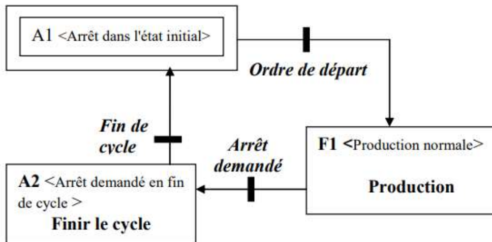
Figure 2.14 : GEMMA d'une machine avec arrêt normal en fin de cycle.
