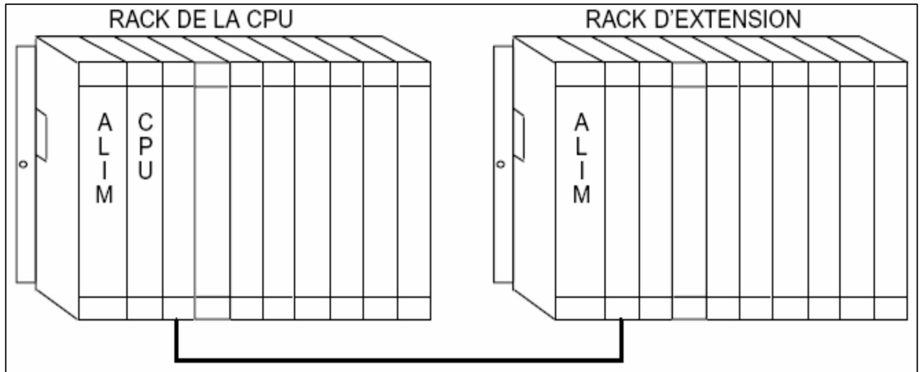
Figure 1-21: Exemple d'implantation de modules dans un API
