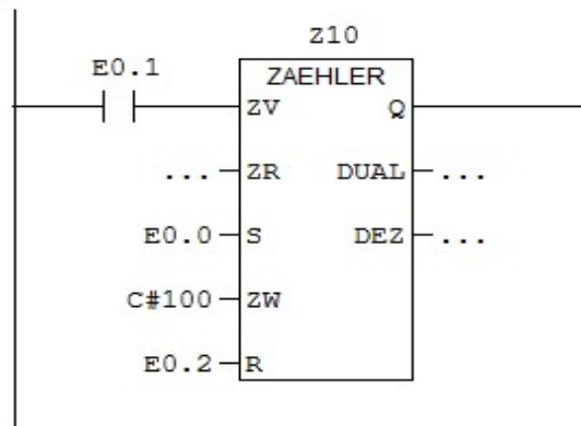
Figure 3- 34: Exemple de programmation d'un compteur
