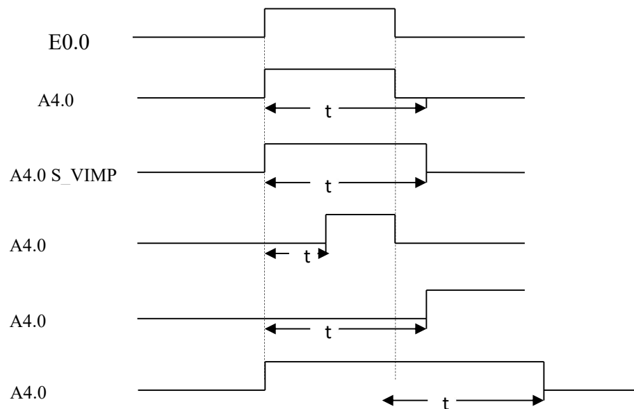
Figure 3- 37: Chronogrammes de fonctionnement des cinq temporisateurs
