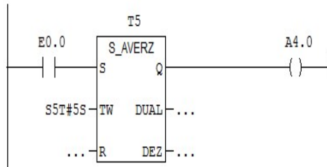
Figure 3- 36: Exemple de programmation des temporisateurs
