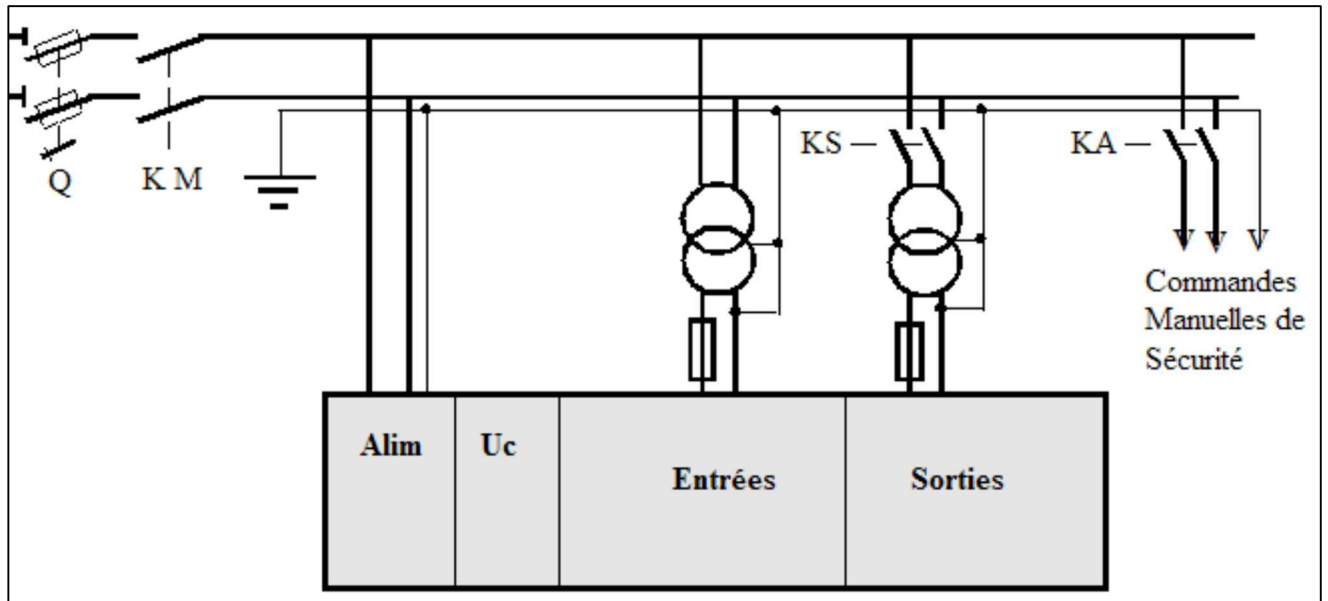
Figure 1-24: Schéma de principe de la mise sous tension du module automate et des entrées
