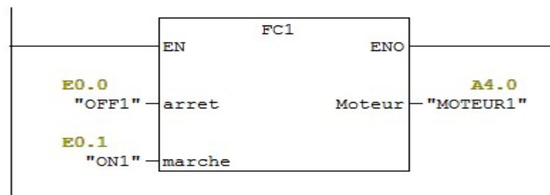
Figure 3- 18: Exemple d'appel à une fonction à partir d'OB1
