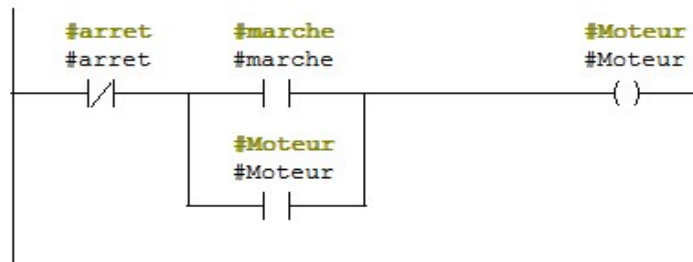
Figure 3- 17: Exemple du contenu d'une fonction
