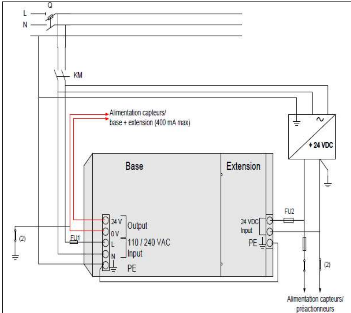
Figure 1-26: Schéma de raccordement d'un automate
