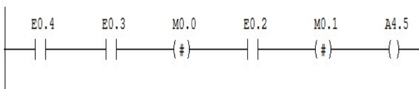
Figure 3- 23: Exemple d'utilisation de la fonction inverser RLG
