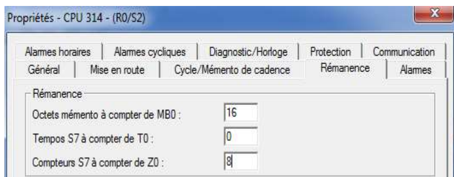
Figure 3- 8: Zones de rémanence de la CPU 314
