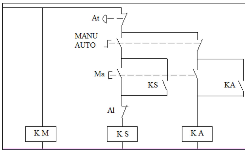
Figure 1-25: Schéma de principe de la mise sous tension des sorties ou des commandes manuelles de sécurité.
