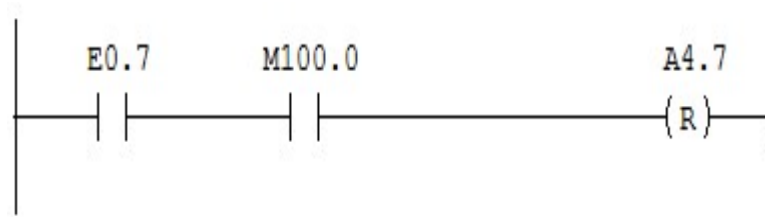
Figure 3- 51: Programme de désarmement du blocage du système
