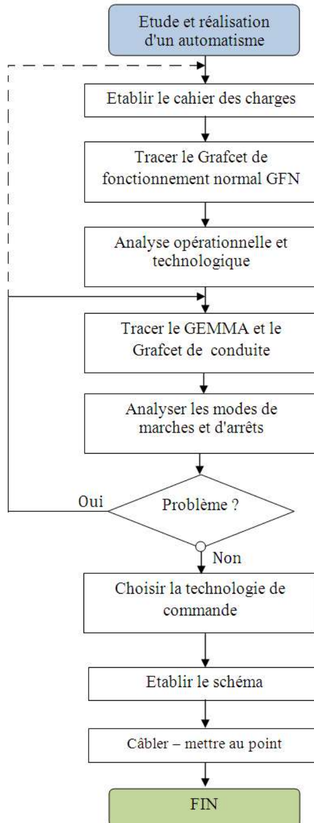
Figure 2-1: Organigramme de Conception d'un automate séquentiel
