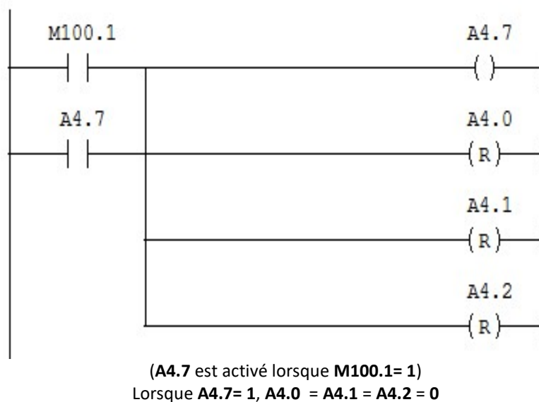
Figure 3- 50: Programme d'activation du voyant NB_D
