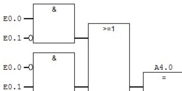
Figure 1-16: Exemple de programme écrit en langage logigramme
