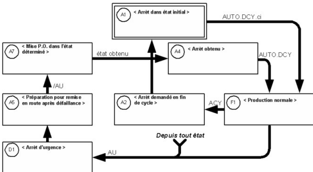
Figure 2.16 : GEMMA d'une machine avec arrêt d'urgence et remise en route à l'état où la machine était lors de l'arrêt d'urgence.
