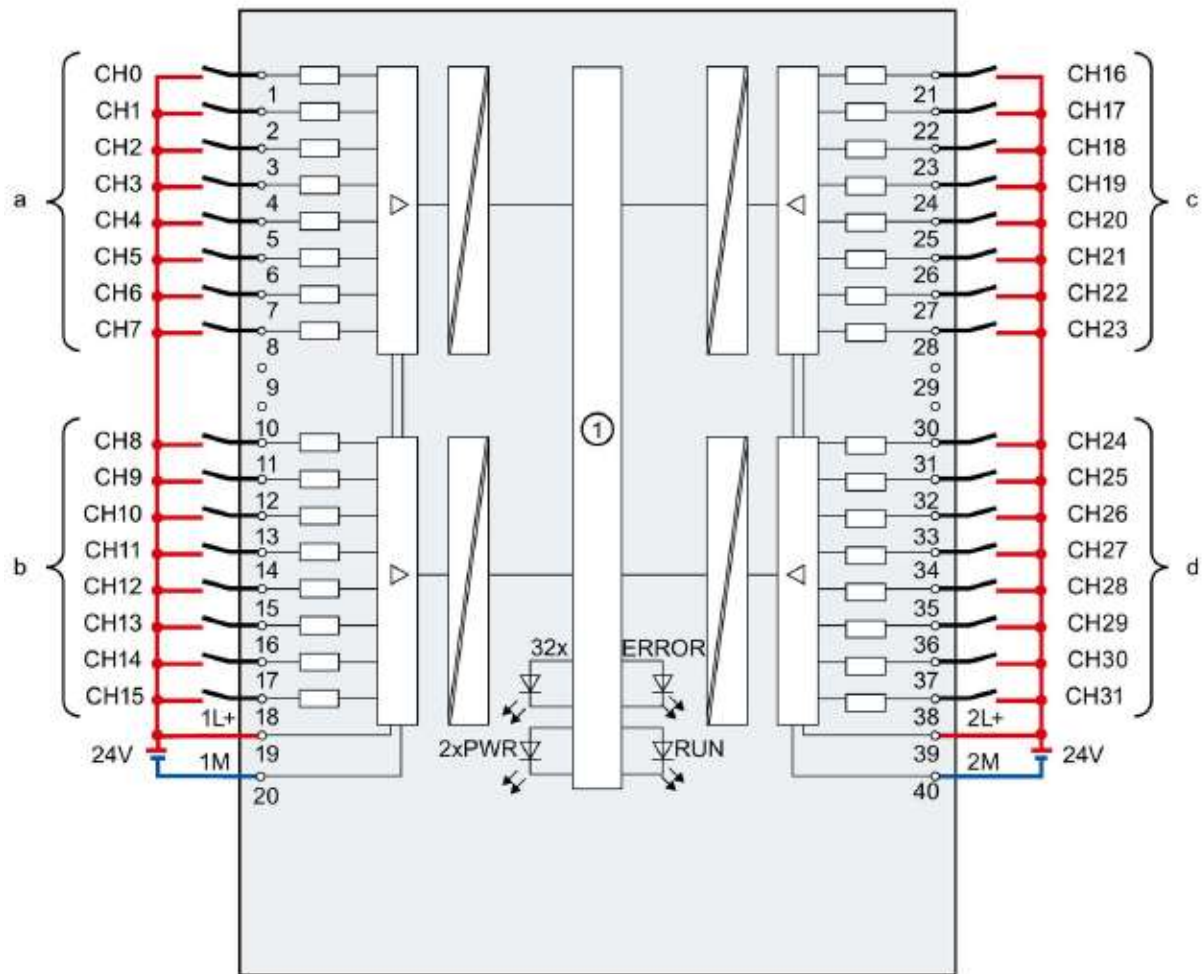
Figure 1.32 : Schéma de câblage d'un module d'entrée logique - Module 32DI (6ES7 521 1BL00 0AB0)
