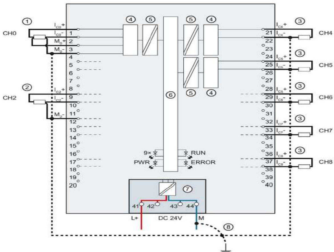
Figure 1.38 : Schéma de câblage d'un module 8AI (6ES7 531 7PF00 0AB0).
