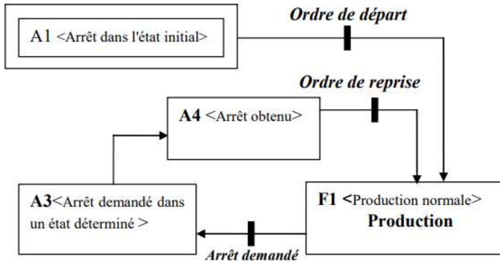
Figure 2.13 : GEMMA d'une machine avec arrêt normal en cours de cycle.
