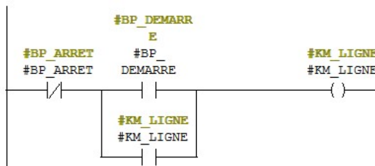
Figure 3- 41: Réseau de commande du contacteur de ligne (KM_Ligne)
