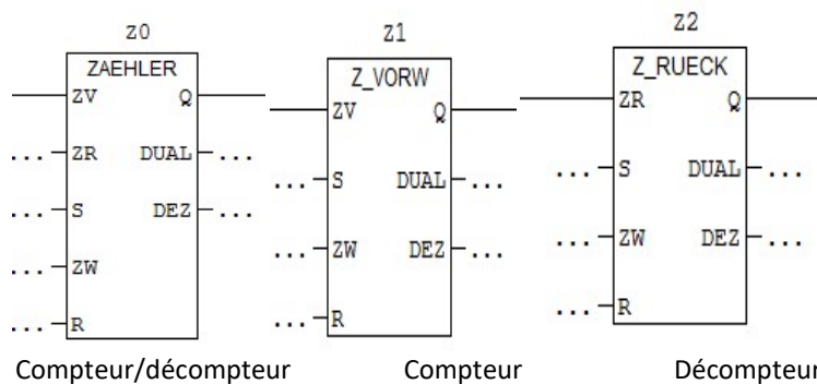
Figure 3- 33: Représentation allemande des compteurs
