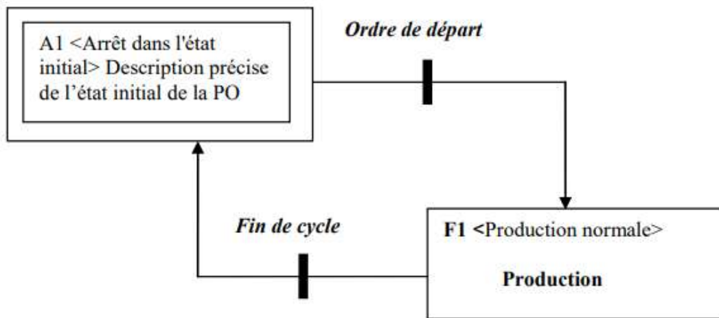
Figure 2.9 : GEMMA d'une machine avec marche de production cycle par cycle.
