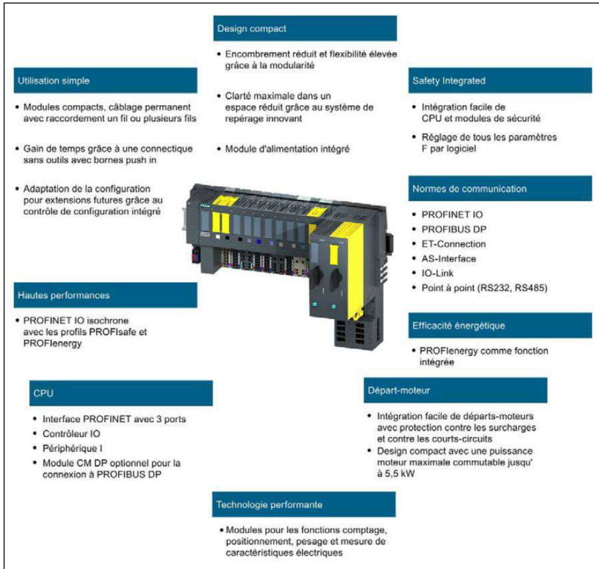
Figure 1.31 : Caractéristiques techniques du module déporté ET 200SP
