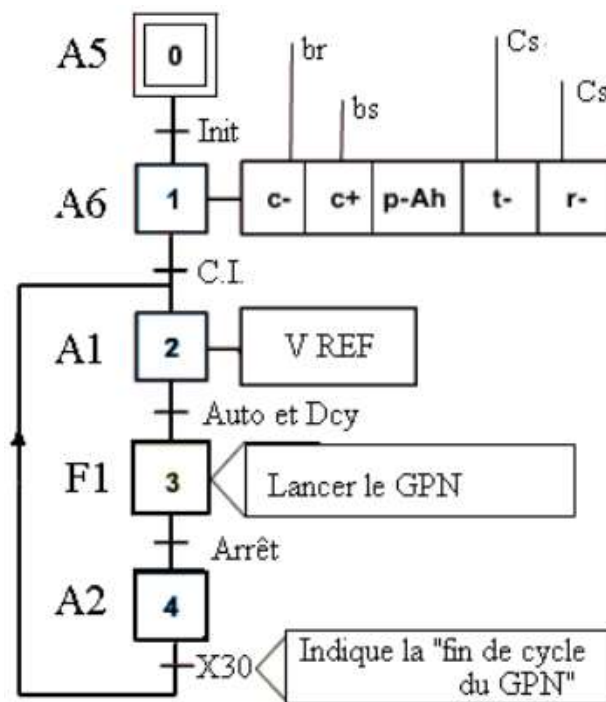
Figure 2.23 : GRAFCET de conduite déduit du GEMMA de la figure précédente.
