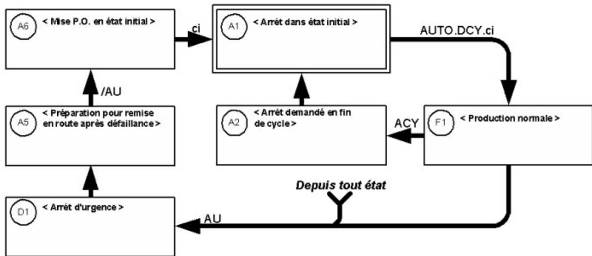
Figure 2.15 : GEMMA d'une machine avec arrêt d'urgence
