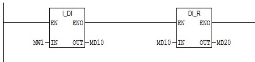
Figure 3- 28: Exemple de programmation d'une conversion nombre entier → nombre réel
