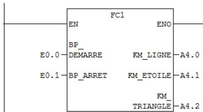
Figure 3- 44: Appel de la fonction FC1
