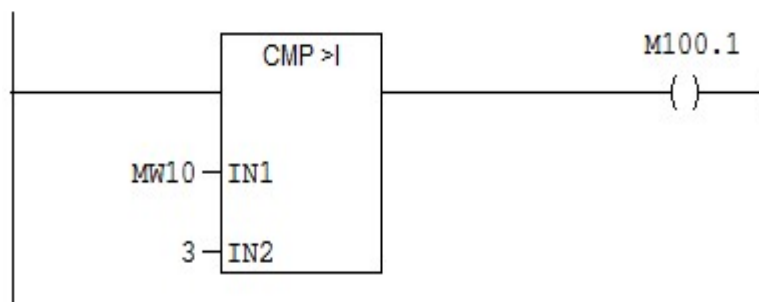
Figure 3- 49: Programme de comparaison du nombre de démarrage à 3
