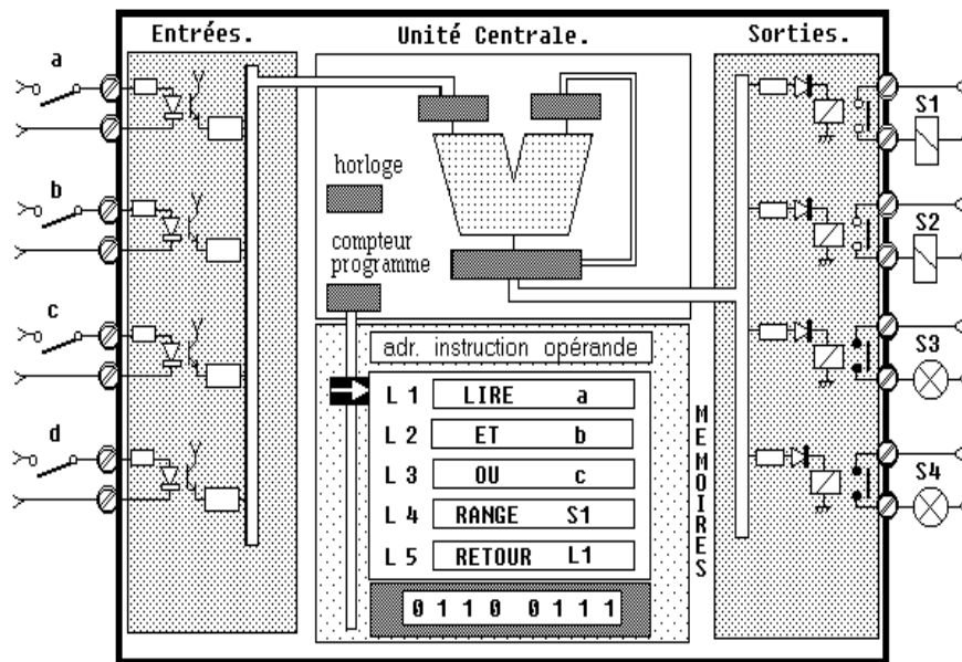
Figure 1 .7 : Eléments de base d'un API
