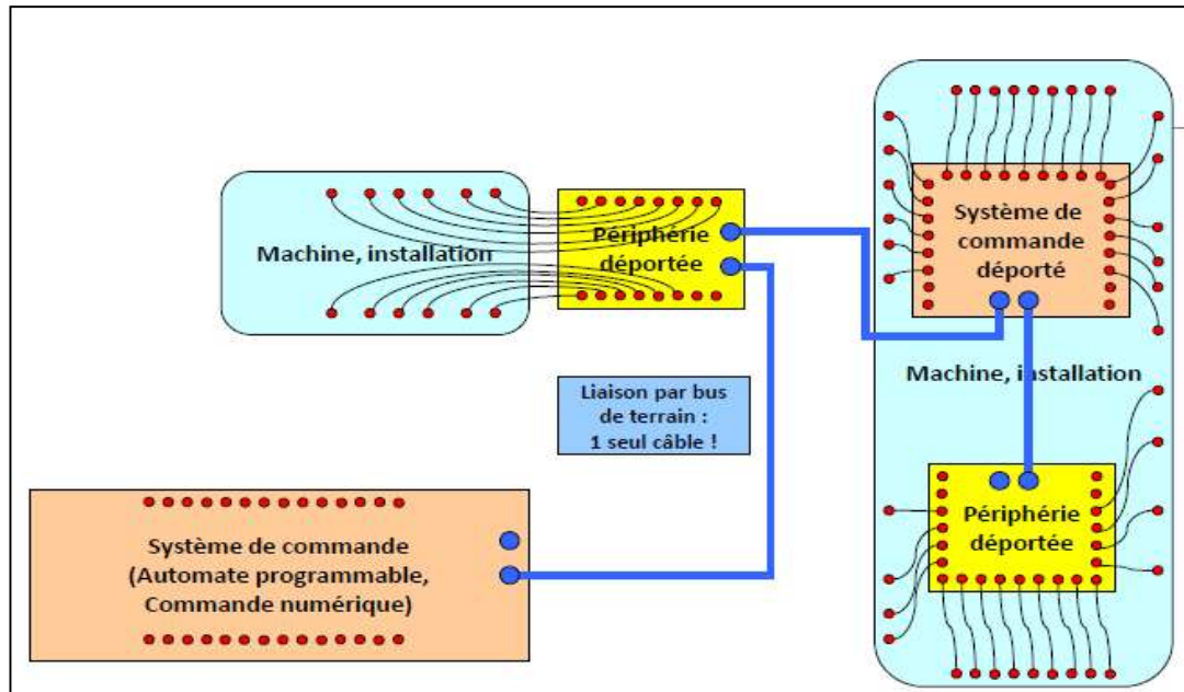
Figure 1 .5 : Schéma de principe d'une architecture décentralisée
