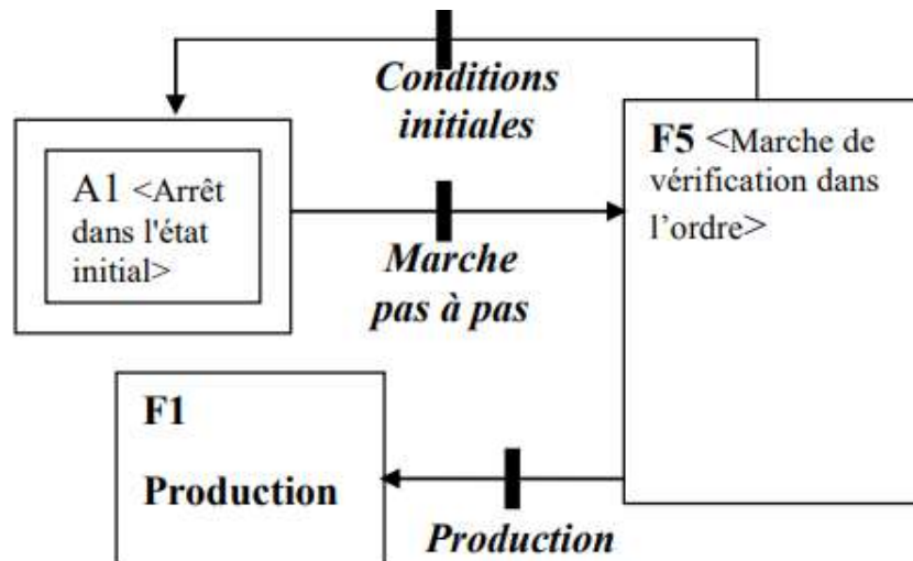
Figure 2.11 : GEMMA d'une machine avec marche de vérification dans l'ordre de cycle.
