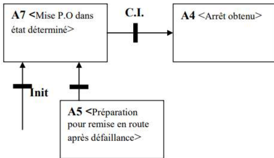
Figure 2.18 : GEMMA d'une machine avec redémarrage à l'étape initiale.
