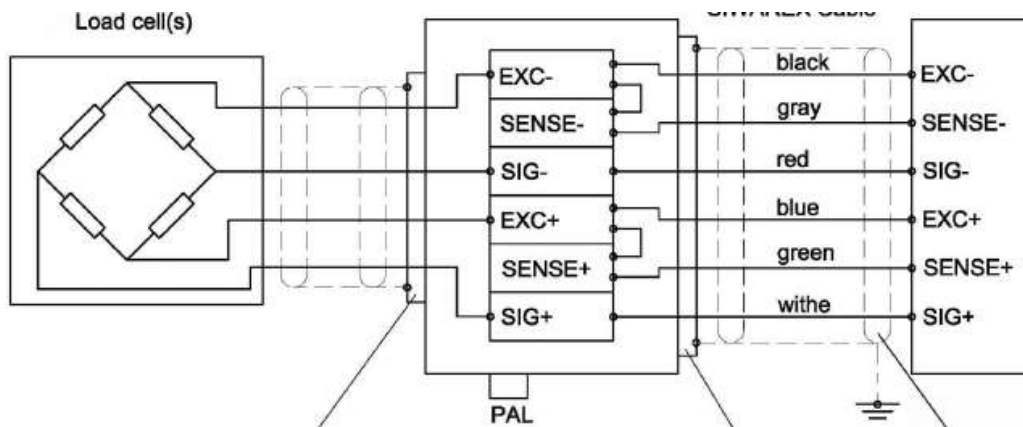
Figure 1.41 : Schéma de câblage du module TM SIWAREX WP521 ST (7MH4 980 1AA01).
