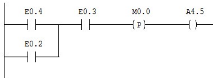
Figure 3- 25: Exemple d'utilisation de la fonction détecter front montant
