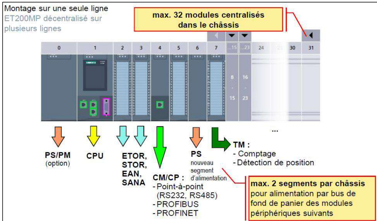
Figure 1.28 : Architecture de l'API S7-1500
