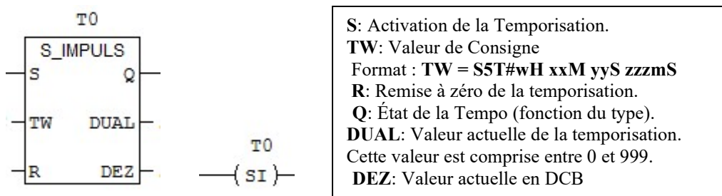
Figure 3- 35: représentation d'une temporisation
