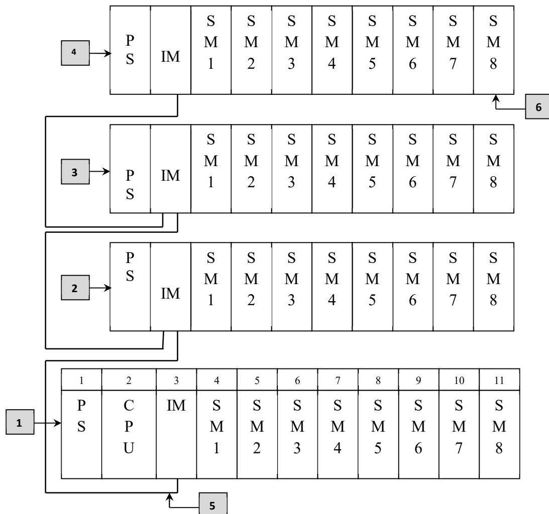
Figure 3- 2 : Disposition des modules dans un montage sur 4 châssis
