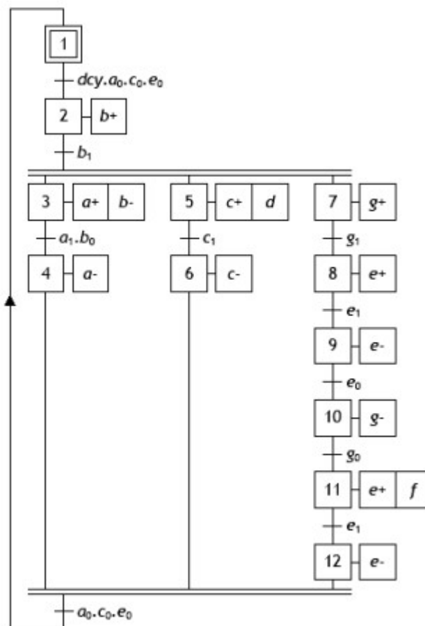
Figure 2.21 : (Grafcet niveau 2) de la Machine à remplir et à boucher
