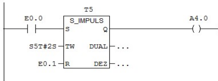
Figure 3- 38: Exemple de programmation d'un temporisateur S_IMPULS
