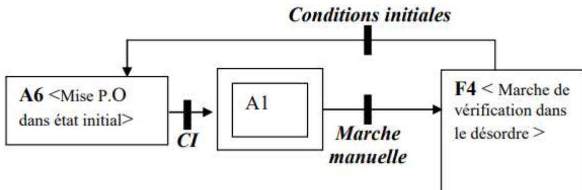
Figure 2.12 : GEMMA d'une machine avec marche de vérification dans le désordre.
