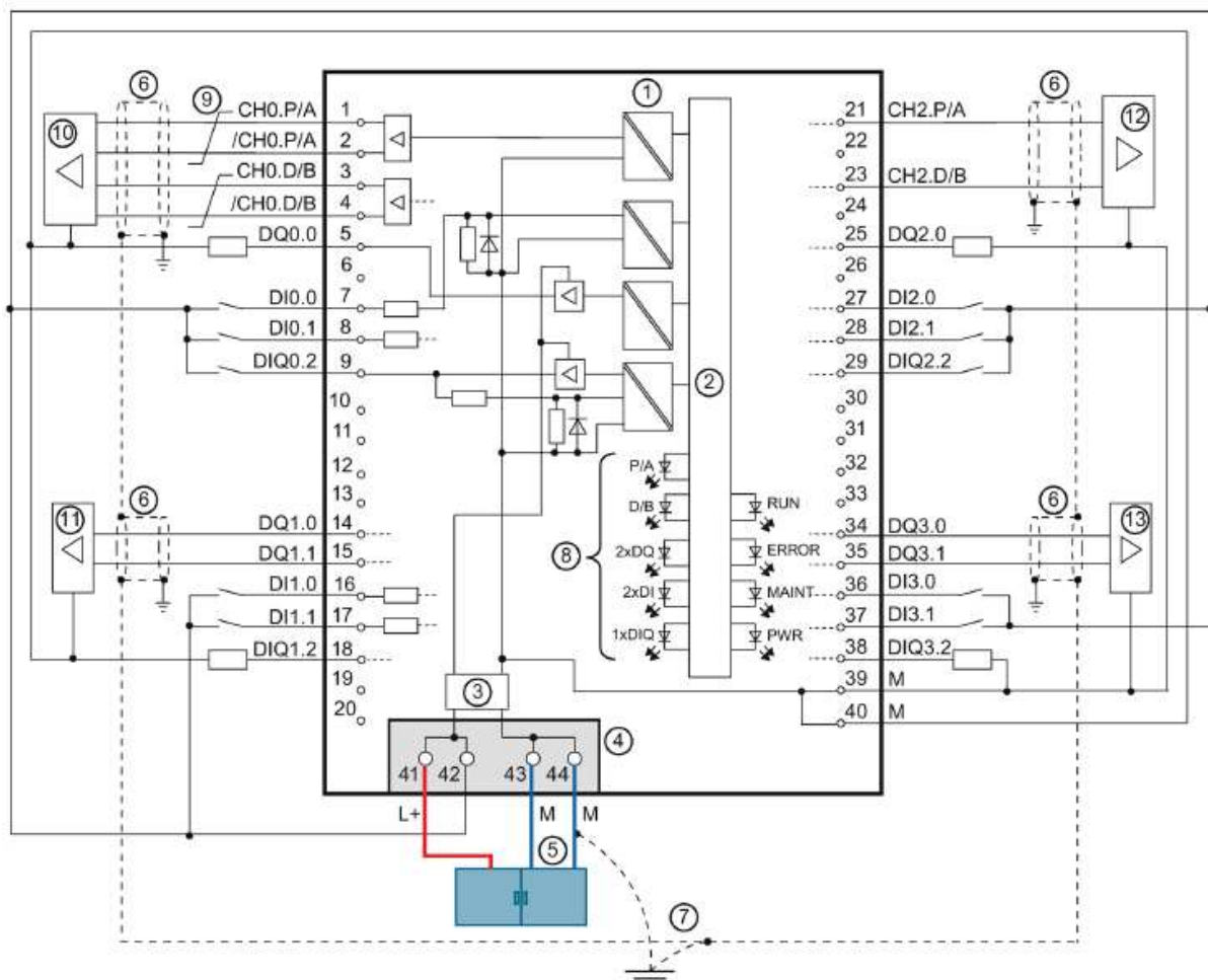
Figure 1.40 : Schéma de câblage du module TM PTO 4 (6ES7 553 1AA00 0AB0).
