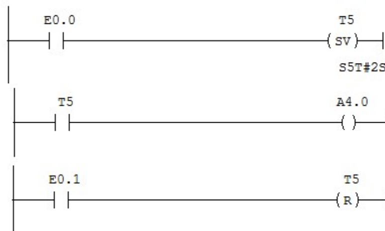
Figure 3- 39: Exemple de programmation d'un temporisateur SV
