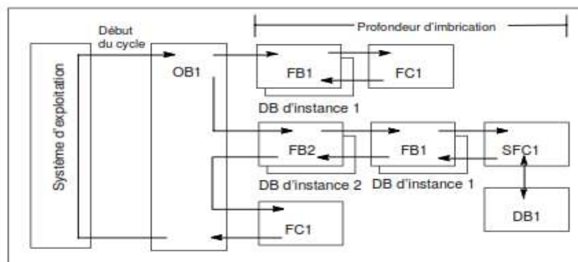
Figure 3- 11: Exemple d'hierarchie d'appel des blocs fonctionnels dans un cycle de traitement.
