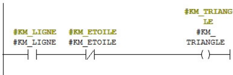
Figure 3- 43: Réseau de commande du contacteur (KM_Triangle)
