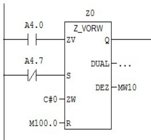
Figure 3- 46: Programme de comptage du nombre de démarrage
