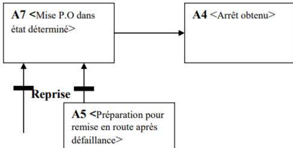
Figure 2.17 : GEMMA d'une machine avec redémarrage à l'étape d'arrêt
