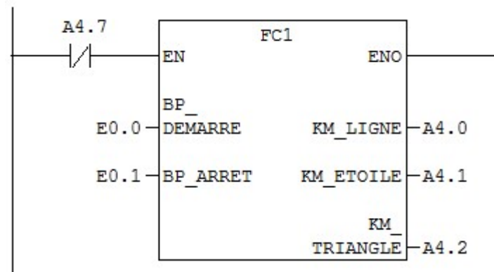
Figure 3- 45: Appel de la fonction FC1 conditionné par A4.7
