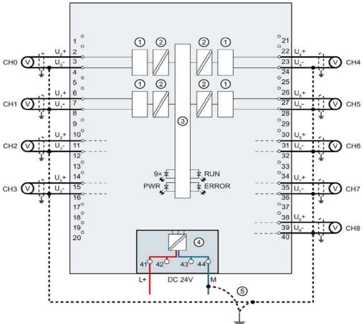
Figure 1.36 : Schéma de câblage d'un module d'entrée analogique - Module 8AI (6ES7 531 7PF00 0AB0)
