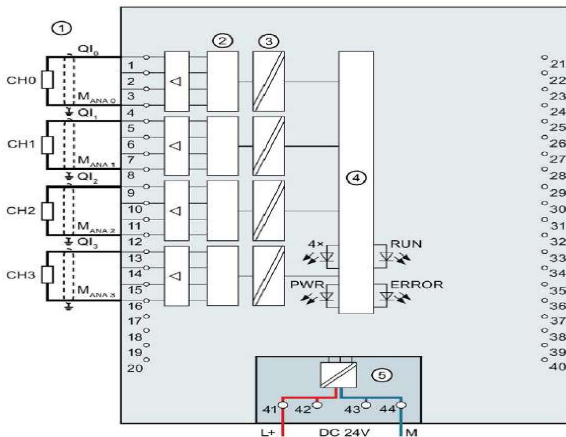
Figure 1.37 : Schéma de câblage d'un module de sortie analogique - Module 4AQ (6ES7 532 5ND00 0AB0)
