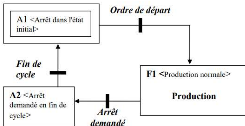
Figure 2.8 : GEMMA d'une machine avec marche de production à cycles répétés
