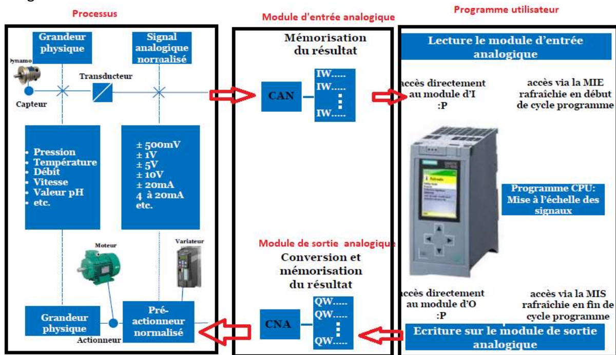
Figure 1.35 : Schéma de principe de traitement des entrées/sorties analogiques
