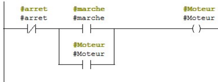
Figure 2- 20: Exemple de contenu d'un bloc fonctionnel
