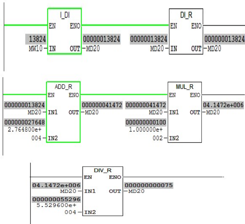
Figure 3- 31: Exemple de programmation d'une mise à l'échelle d'une entrée de type entier en format bipolaire (Résultat de simulation pour MW10 = 13824)
