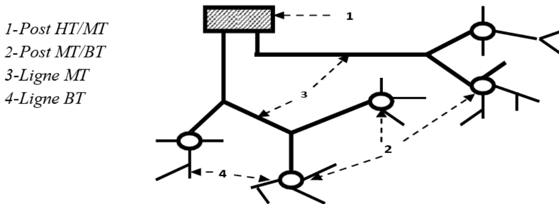
Figure 14.3 : Réseau radial
