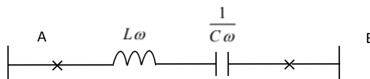
Figure 19.2 : Compensation Série
