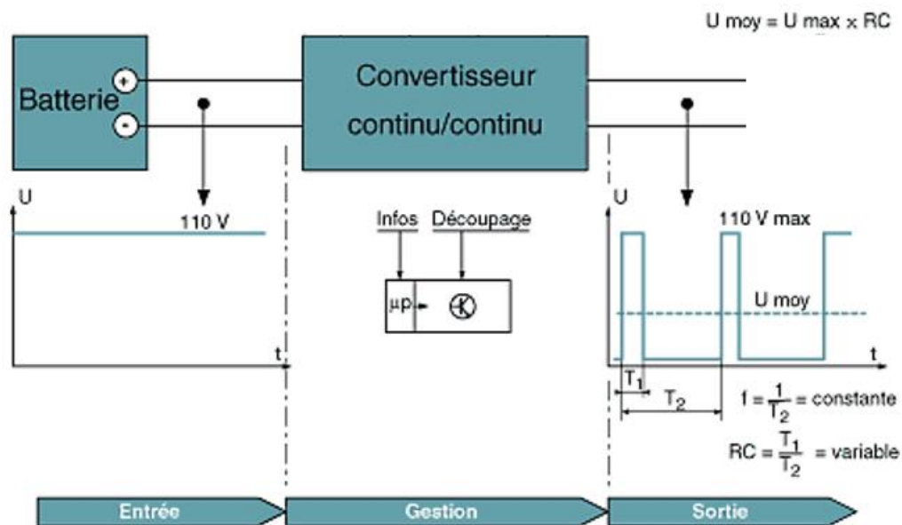
Figure 21.1 : Schéma de fonctionnement d'un hacheur
